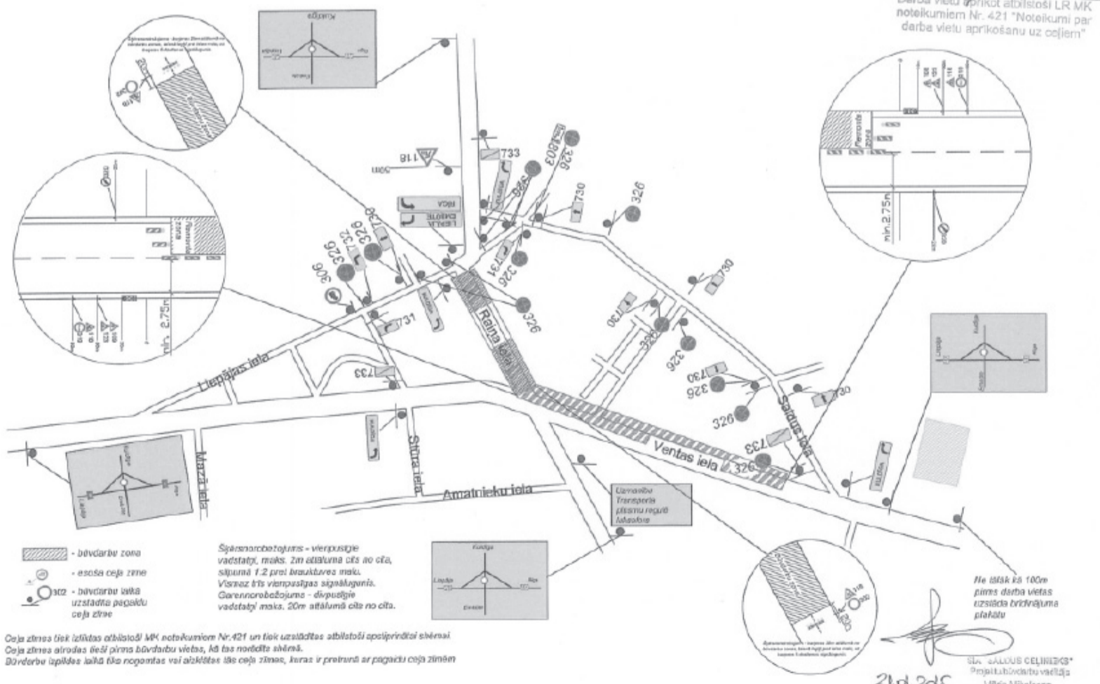
SKRUNDAS PILSĒTAS SATIKSMES ORGANIZĀCIJAS SHĒMA BŪVDARBU LAIKĀ SHĒMA NR.13
