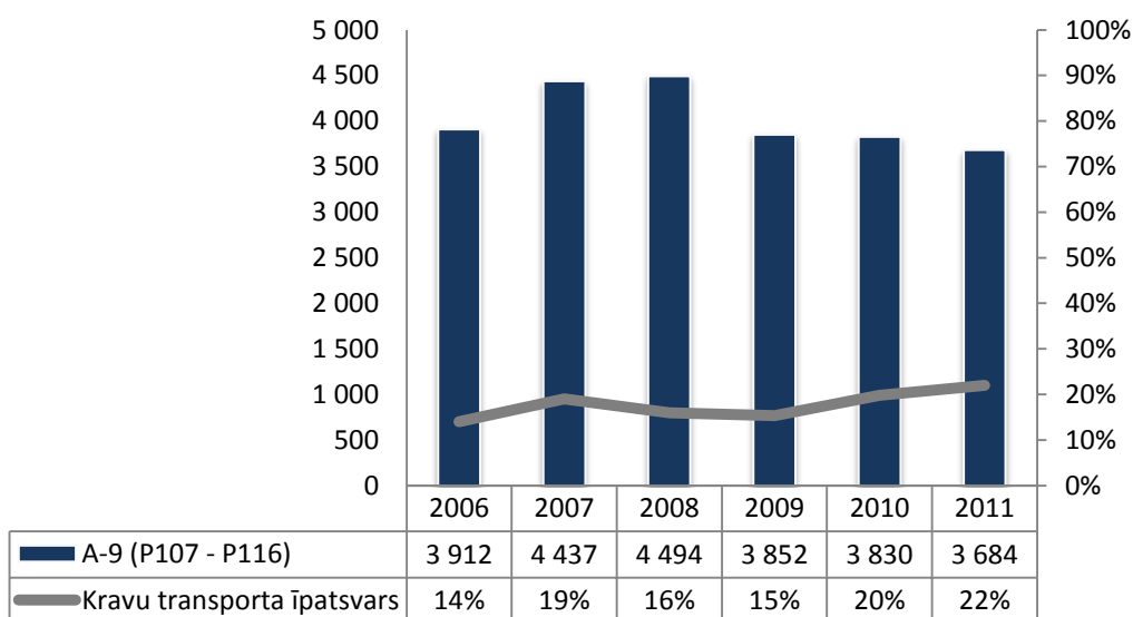
Ilustrācija 5-5. Satiksmes intensitātes dinamika uz valsts galvenā autoceļa A-9 Rīga (Skulte)-Liepāja (P109 – P116)) Skrundas novadā
